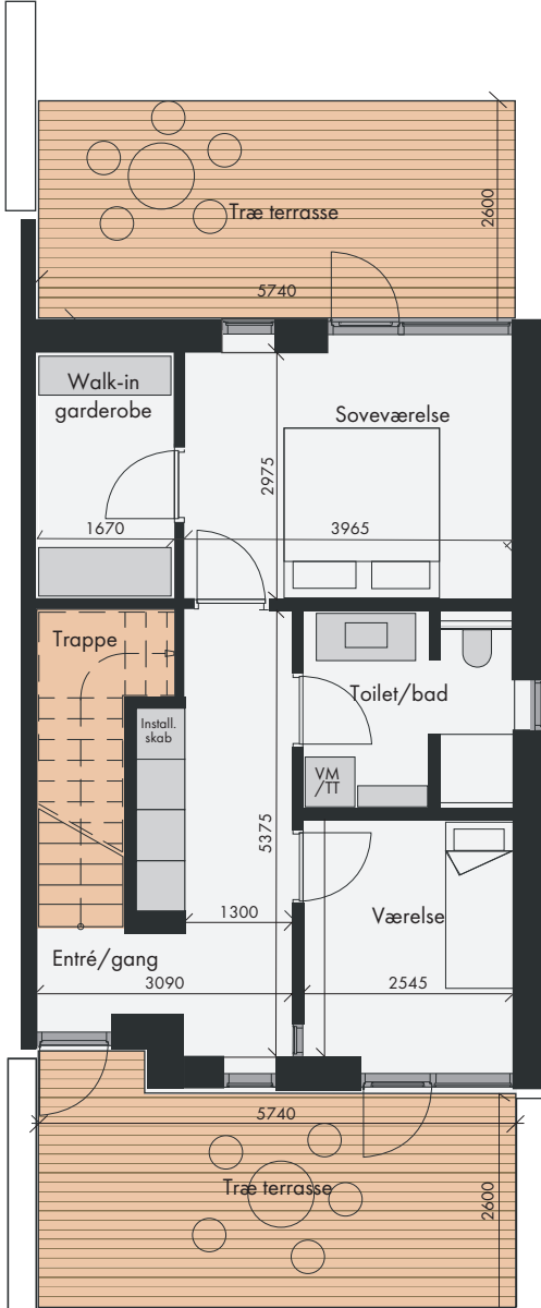
STUEPLAN
