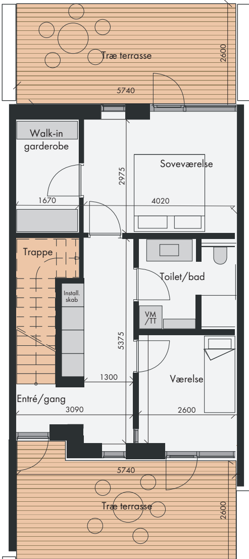
STUEPLAN
