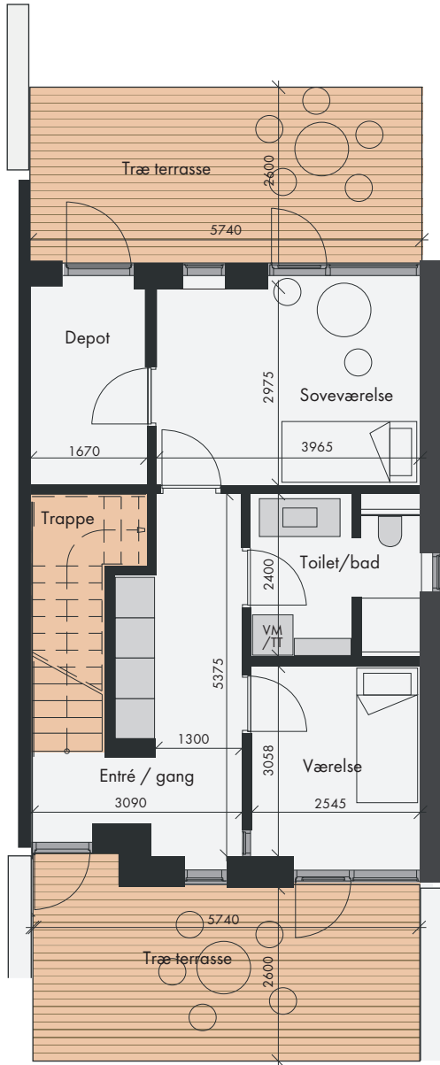
STUEPLAN
